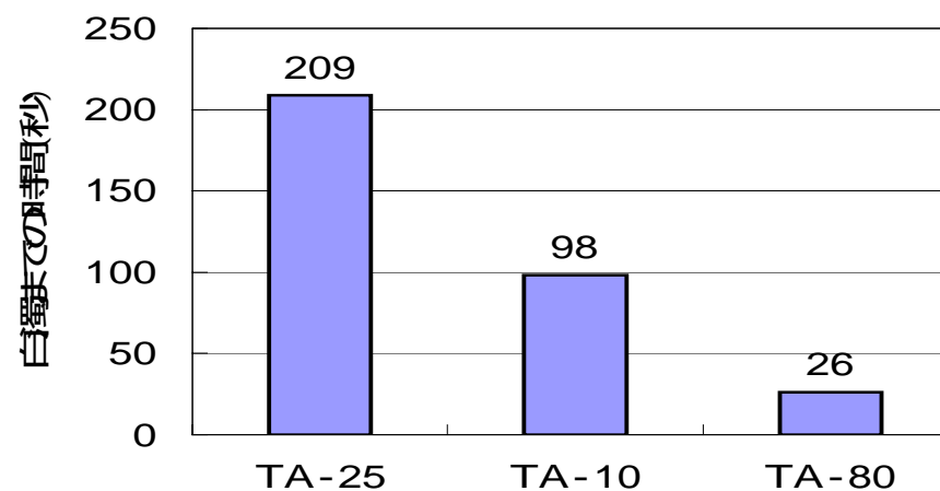
チタンアルコキシドの加水分解速度の比較
