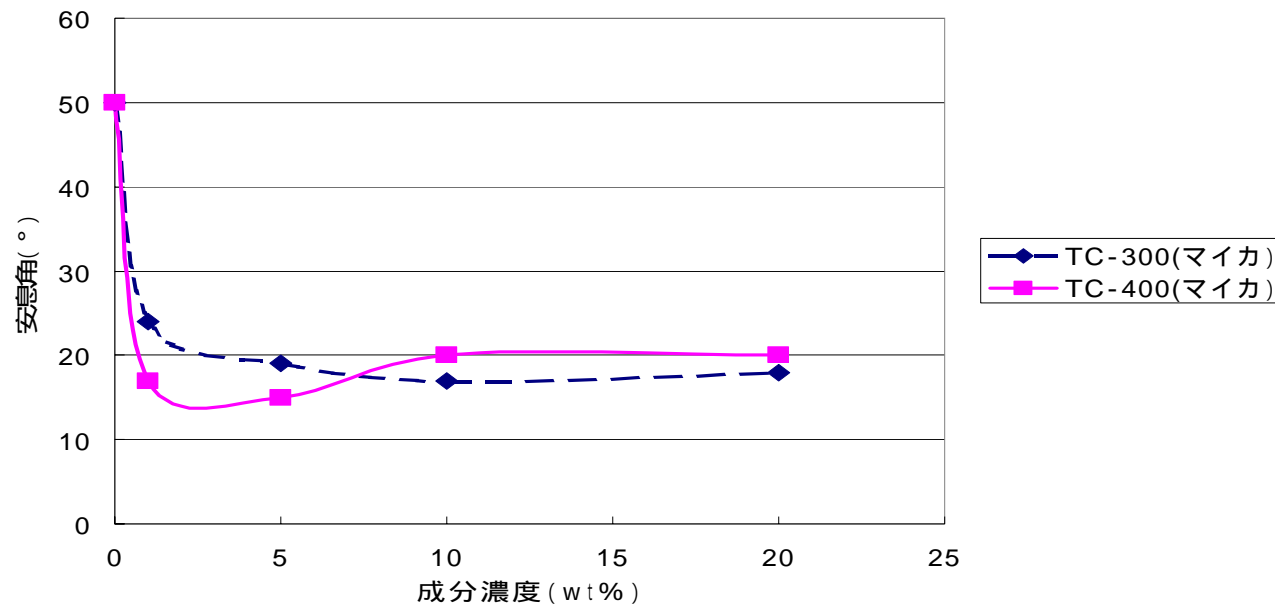
TC-300,TC-400による表面処理:安息角
