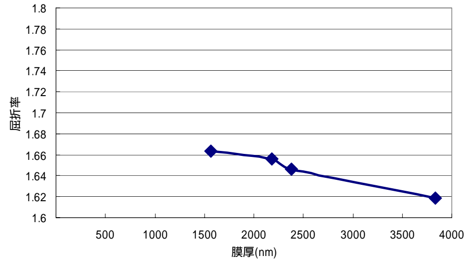
100 30秒乾燥時の膜厚と屈折率の関係
