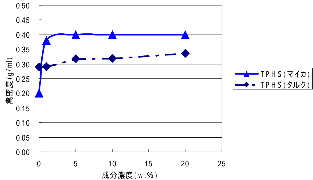
TPHS処理による嵩密度変化
