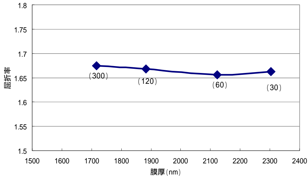
100 乾燥時の(乾燥時間)膜厚と屈折率の関係
